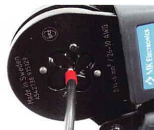
スクエアクリンプ圧着イメージ
