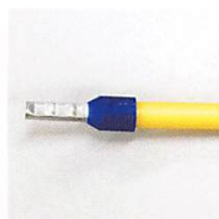
AC25SQT圧着形状
