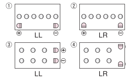
T:テーパー端子 L:L形端子(ボルト締付端子)
